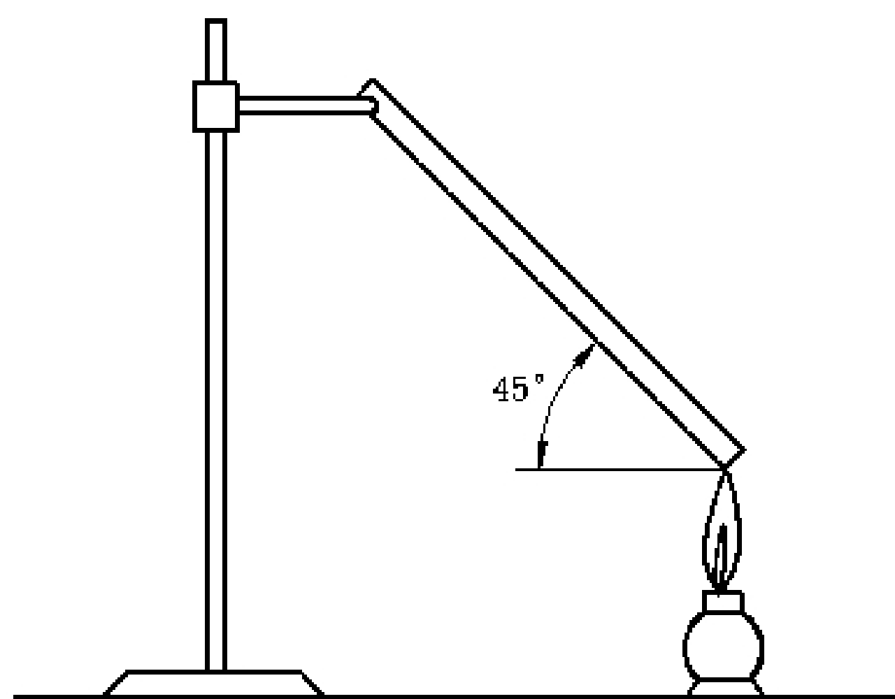
图 4 阻燃性能测试方法示意图
